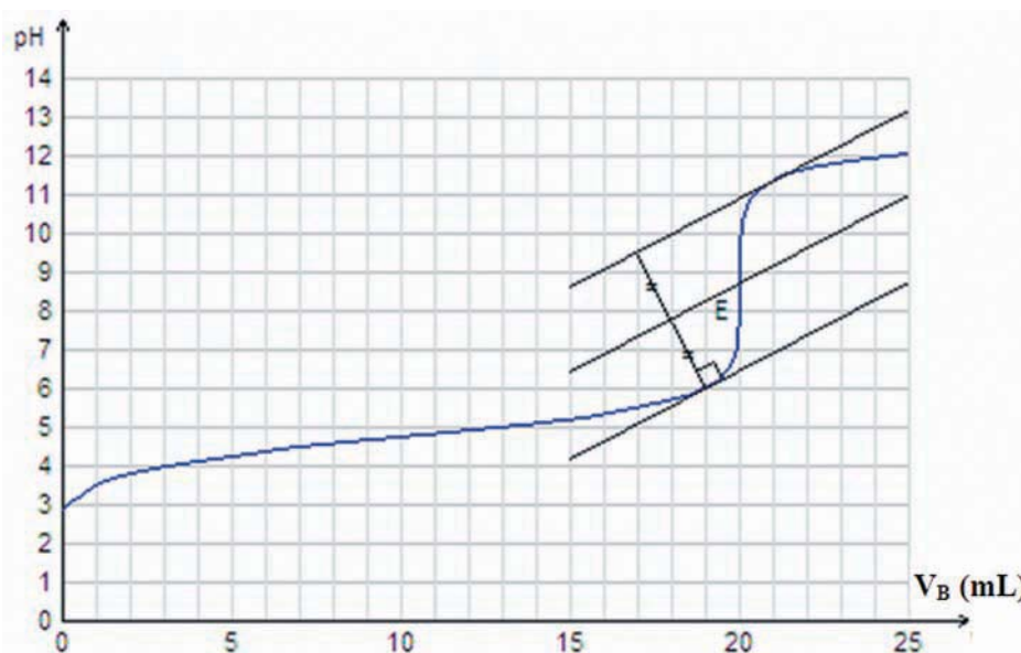
Figure 7. Evolution du pH au cours de l'addition d'une solution aqueuse d'hydroxyde de sodium 10^{-1} M à une solution d'acide éthanóïque 10^{-1} M.
