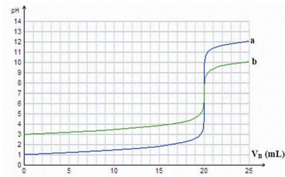
Figure 6. Variation du pH au cours de l'addition d'une solution aqueuse d'hydroxyde de sodium à une solution d'acide chlorhydrique dans le cas où :
